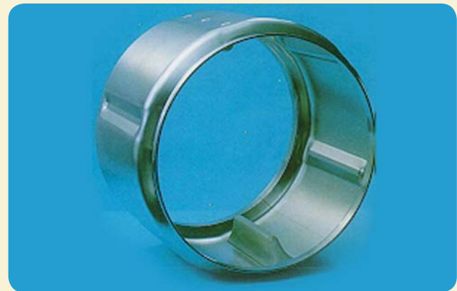
Trocknertrichter, geschweißtes Blech aus 1.4512 (409), expandiert.
